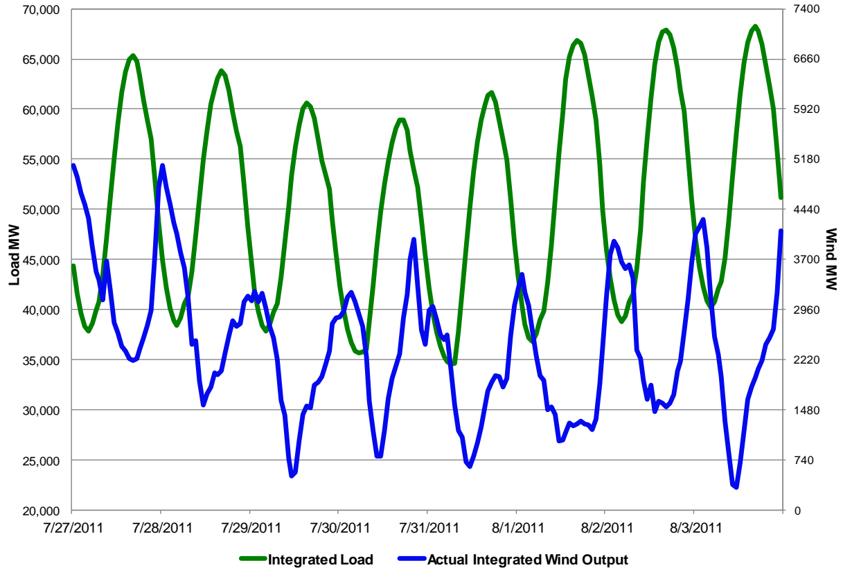
ERCOT Load vs. Actual Wind Output 7/27/2011 - 8/3/2011
