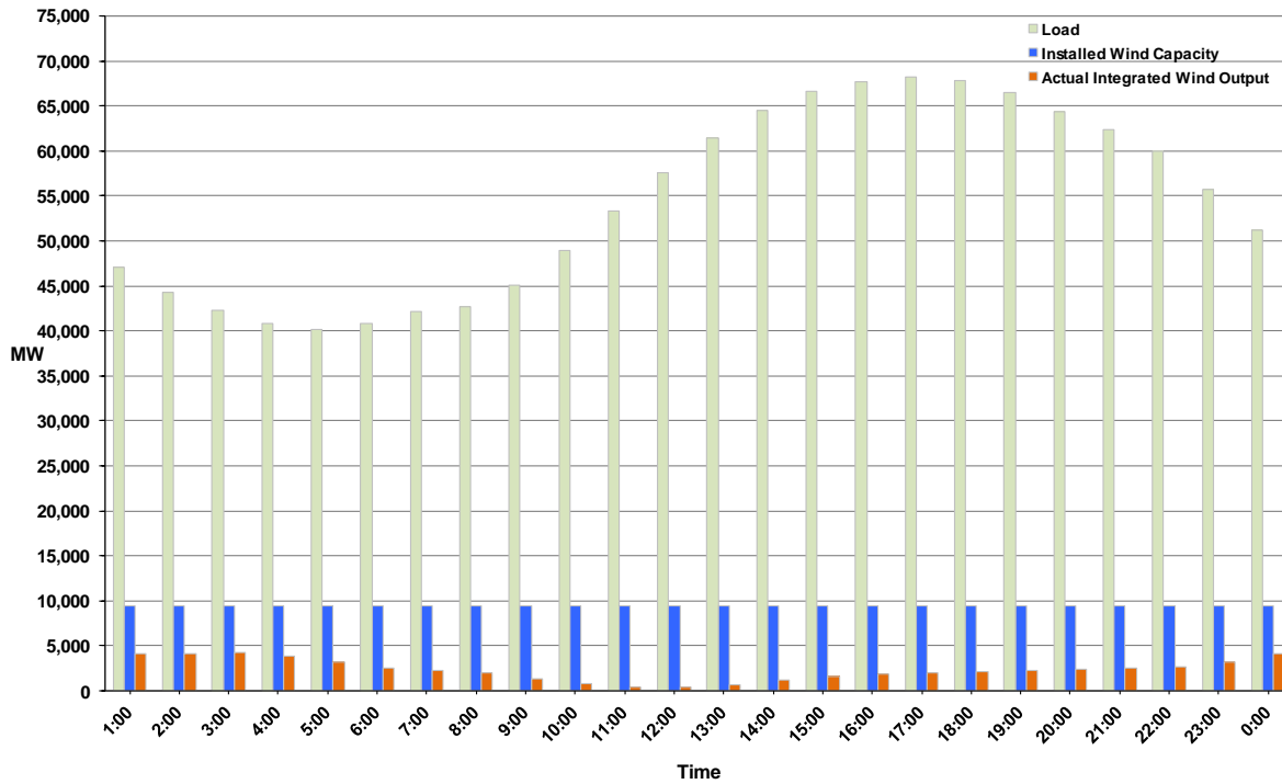
Hourly Average Actual Load vs. Actual Wind Output 08-03-2011
